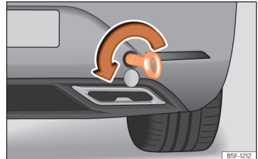
Afb. 214 Aan de rechterzijde van de achterbumper: vastgeschroefd sleepoog.
