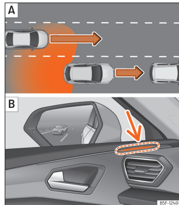
Afb. 145 Schematische weergave: A Inhalen met verkeer aan de achterzijde. B Indicatie van de rijstrookwisselassistent aan de linkerzijde.
