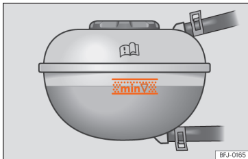
Afb. 221 In de voorruimte: markering aan het koelvloeistofexpansiereservoir.
